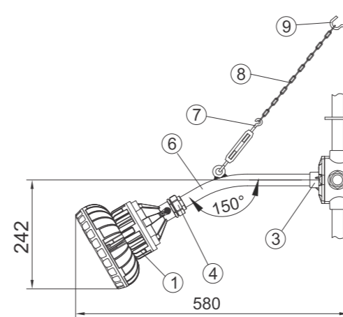
Wall 30°(b1)
